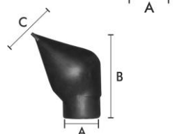
Parte N° DG-4380 VÁLVULA EYECTORA DE POLVO VALVULA EYECTORA DE POLVO ( CP-800-1200-1500)
